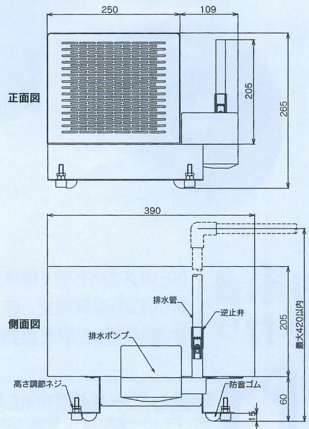
外観図
